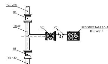
ALZADO
