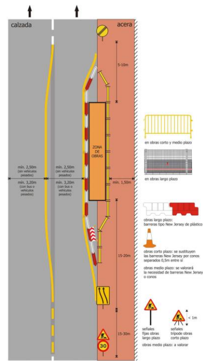
Estrechamiento carril en vía sentido único
