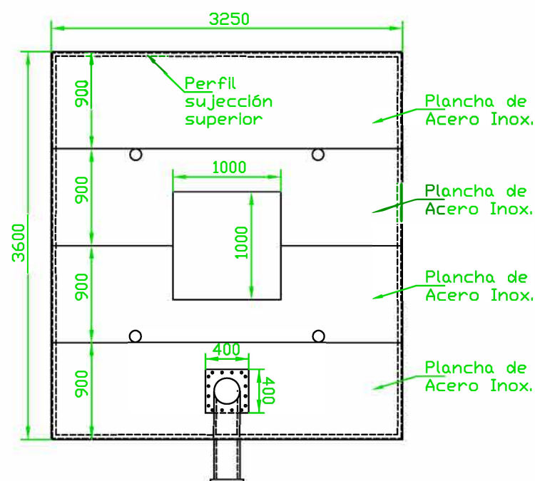
PLANTA POR II
