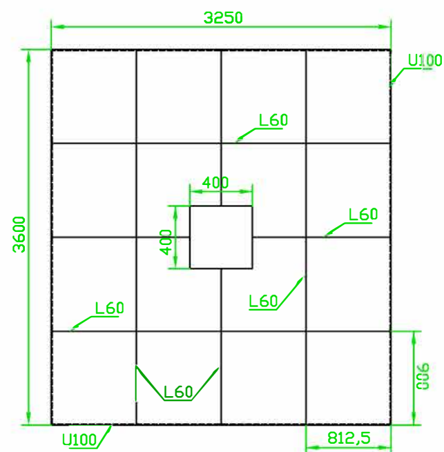
PLANTA POR I
