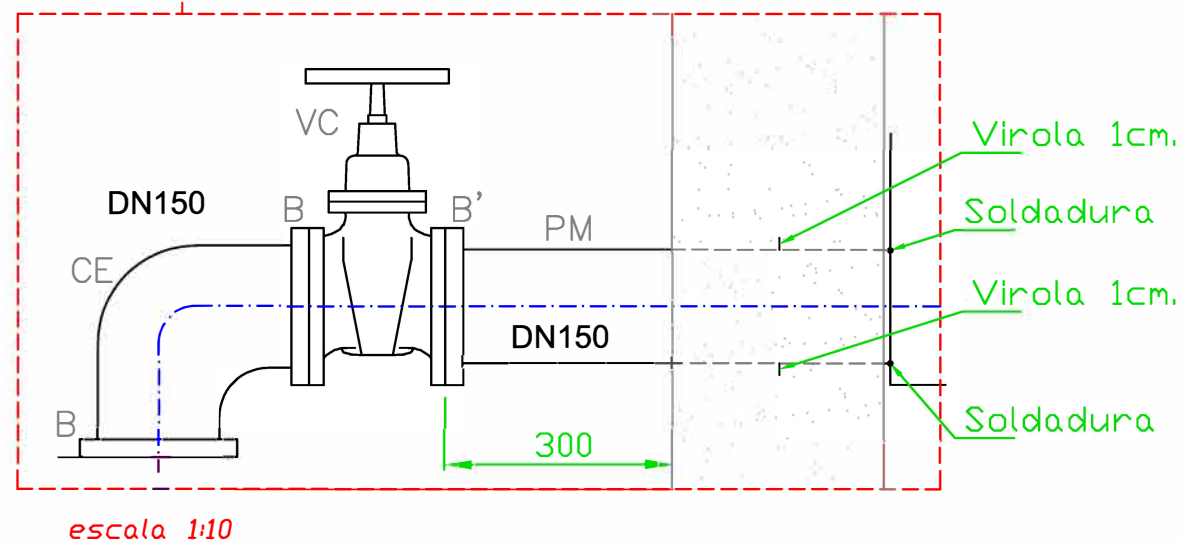
DETALLE VÁLVULA DE FONDO
