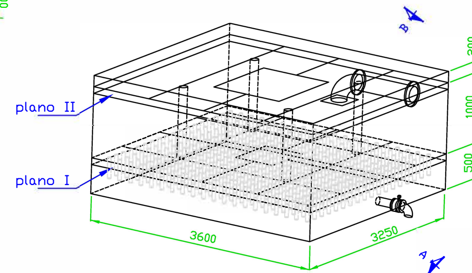
FILTRO DE ARENA
