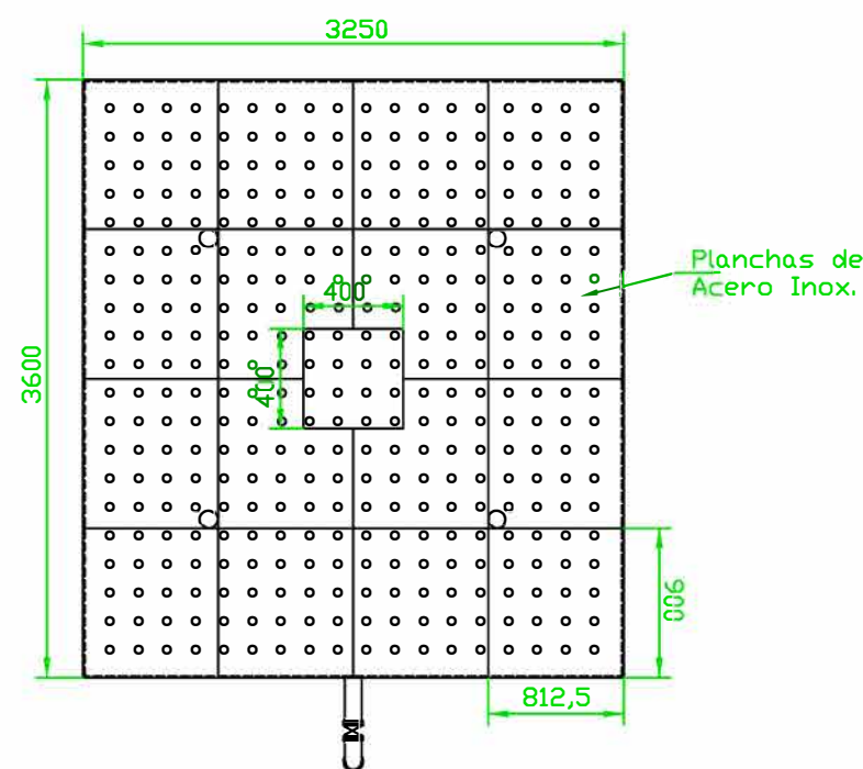
PLANTA POR I
