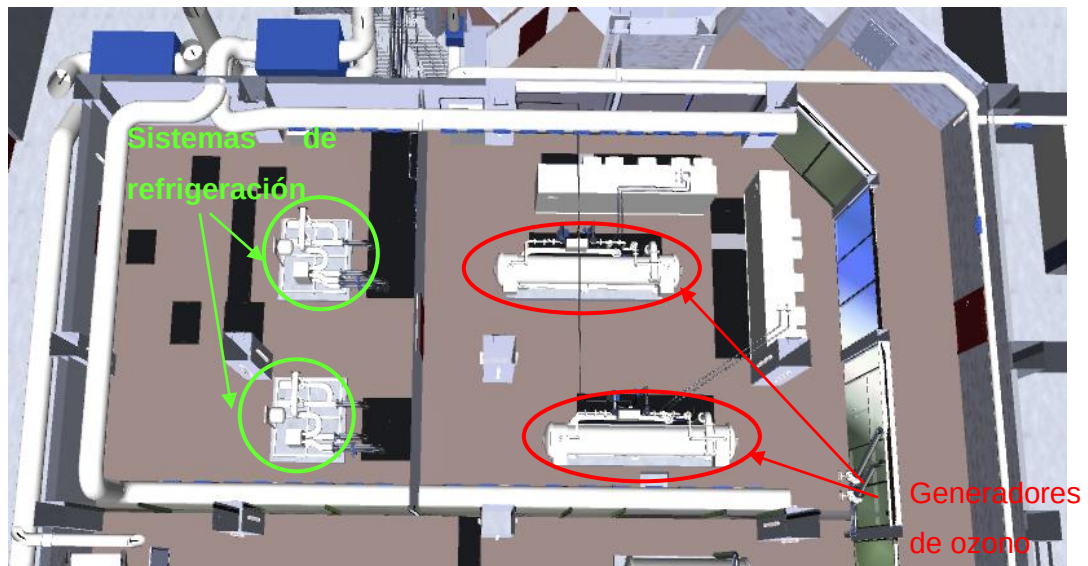
Sala de generación de ozono
