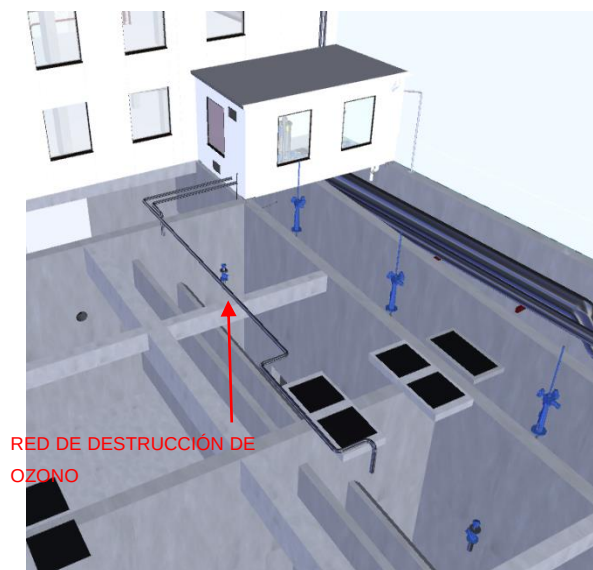
Preozonizacion
