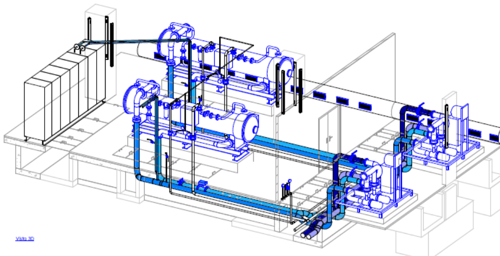
Conexión de agua industrial entre sistemas de refrigeración y generadores de ozono
