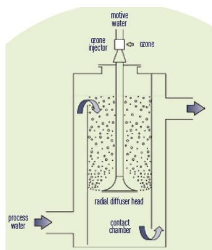
Esquema de funcionamiento de inyección con difusores radiales
