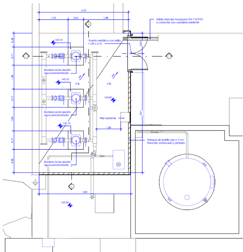
Caseta de bombas proyectada
