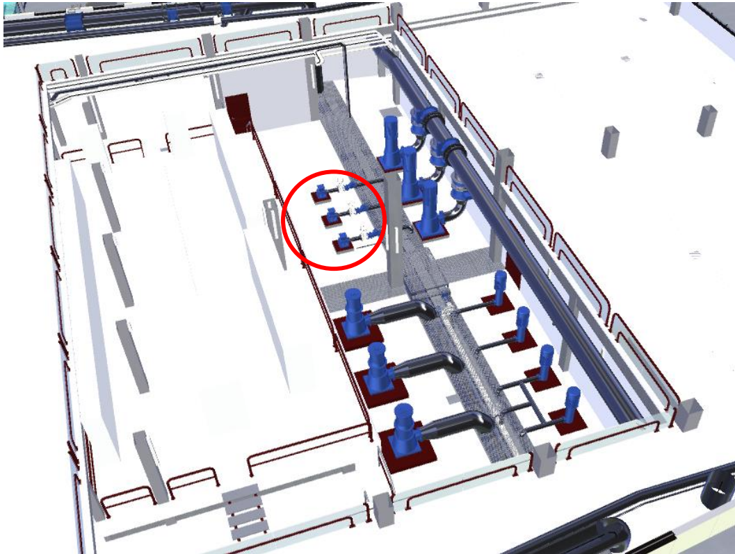
Bombas de agua industrial para sistema de refrigeración y tubería de impulsión
