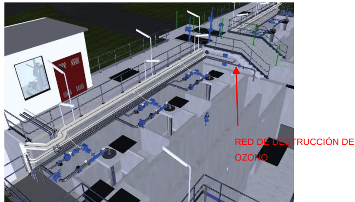
Preozonizacion
