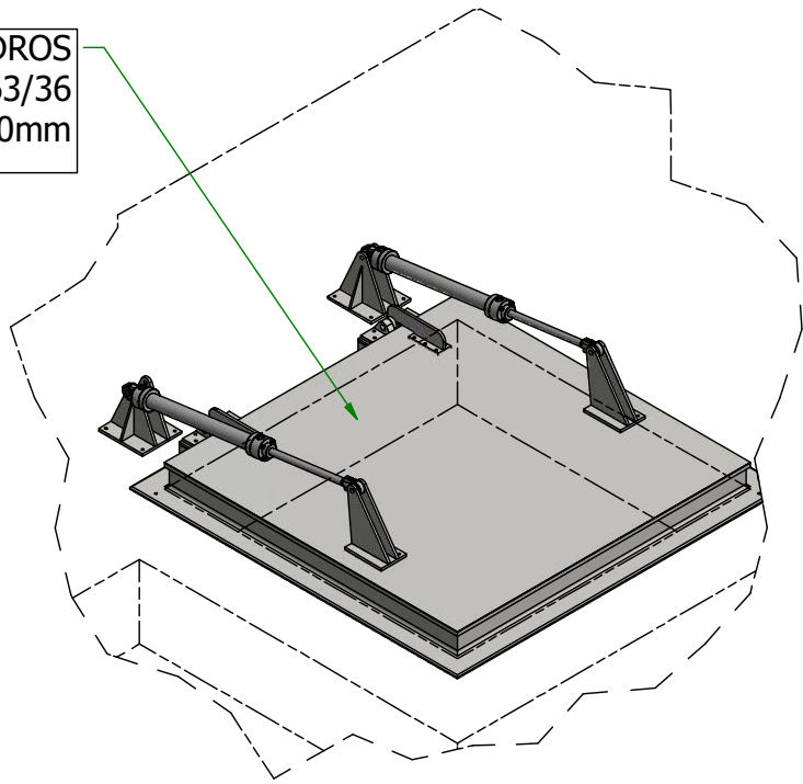
DETALLE A (1 : 40 ) TAPA MANTENIMIENTO
