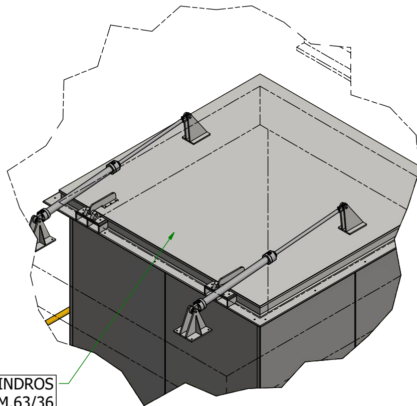
DETALLE B (1 : 40 ) TAPA ENTRADA MATERIAL
