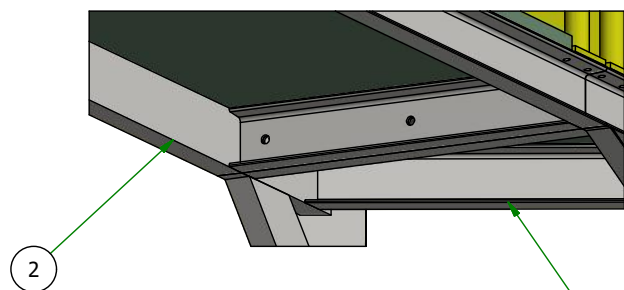
DETALLE UNION ENTRE MODULOS ( 1 : 15 )
