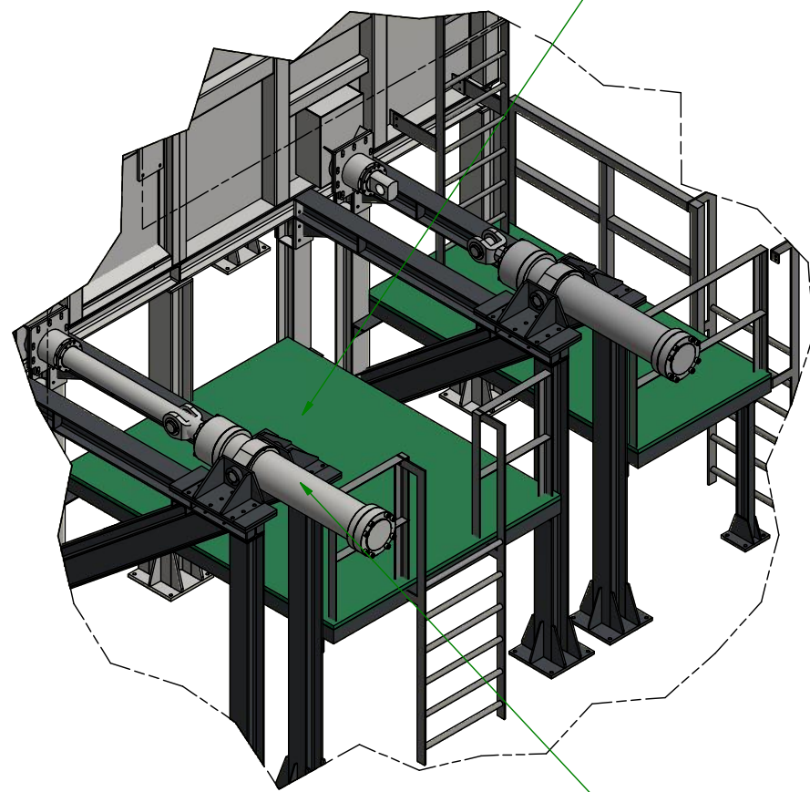
DETALLE C (1 : 40 ) CILINDROS ARRASTRADORES
