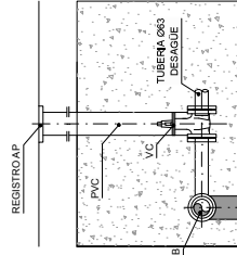
ALZADOC
