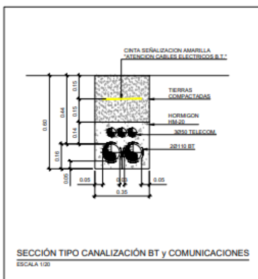
Sección Zanja Tipo
