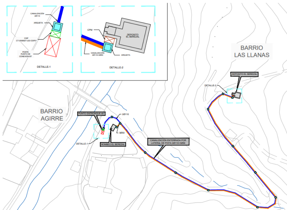
Acometida eléctrica para el Depósito El Berezal
