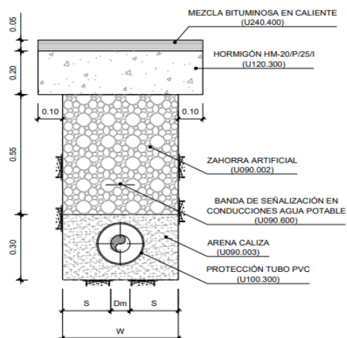
SECCIÓN TIPO CRUCE BAJO INFRAESTRUCTURA LINEAL / Ht ≤ 1,30m/Vertical.
