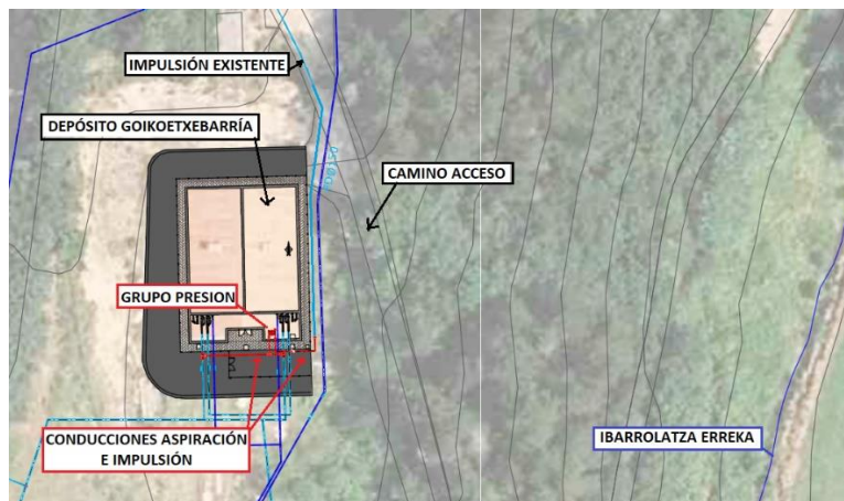
Grupo de presión y conducciones proyectadas
