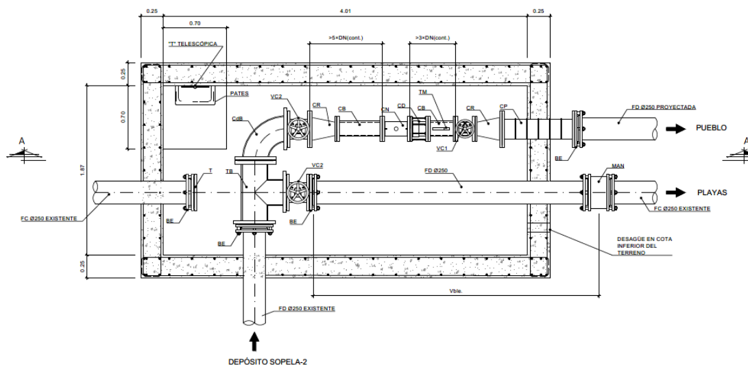
Planta de la arqueta CRE1
