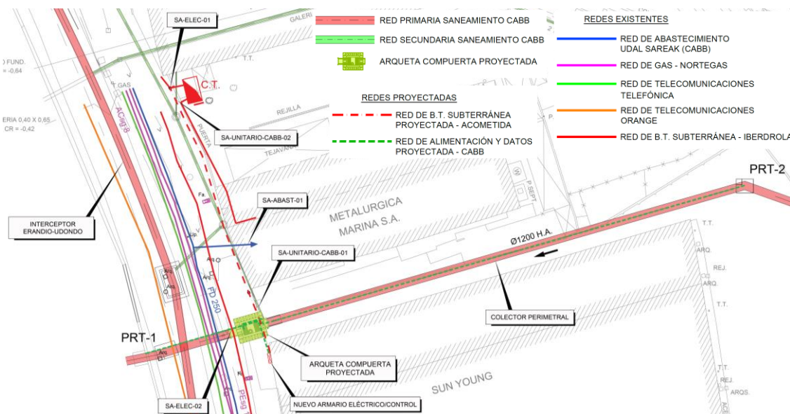
Figura 4. Servicios existentes en la zona de proyecto
