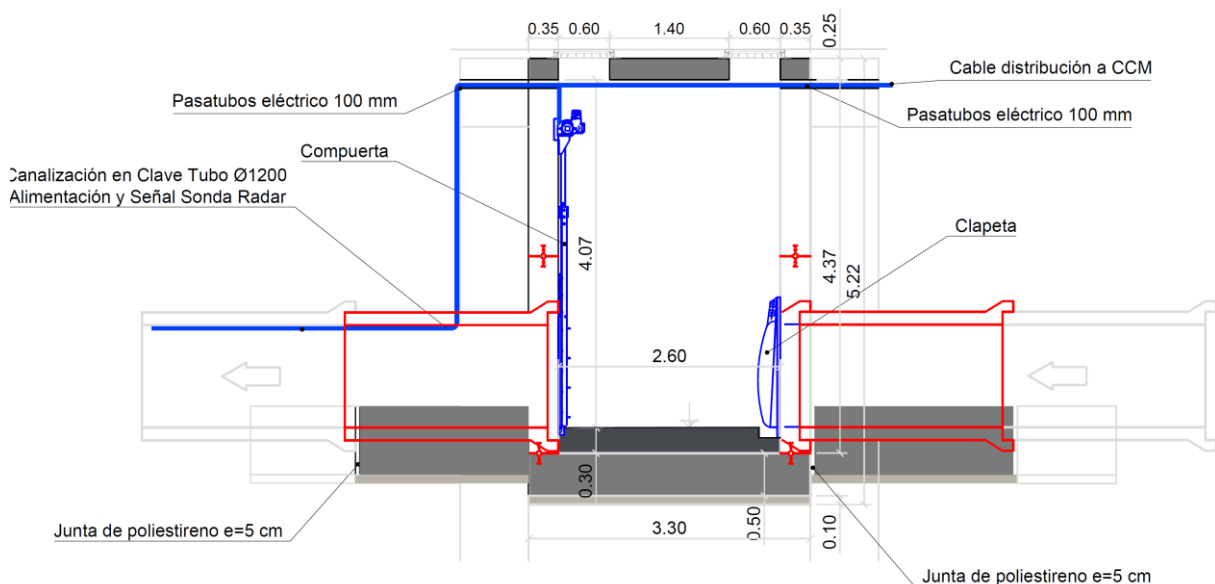
Figura 3. Sección longitudinal de la arqueta proyectada
