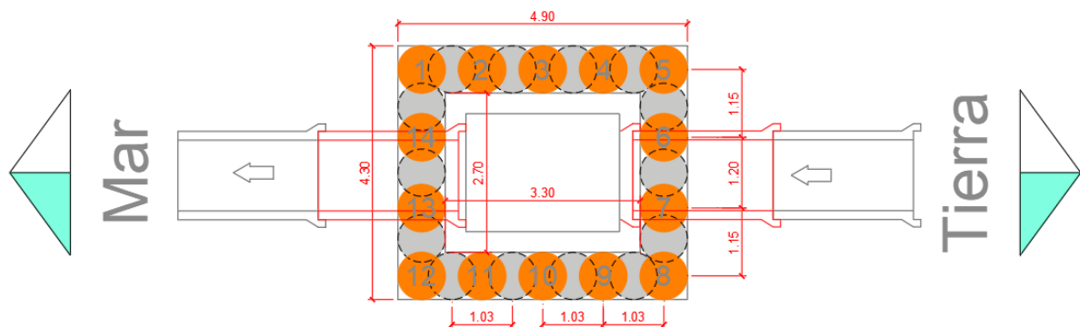
Figura 2. Esquema de las pantallas de pilotes proyectadas
