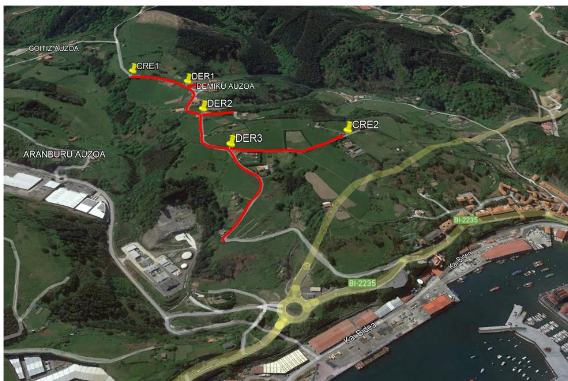
Emplazamiento de la red a reponer en el barrio de Demiku
