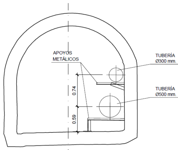
Sección actual intermedia de la galería
