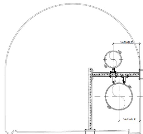
Sección proyectada intermedia de la galería
