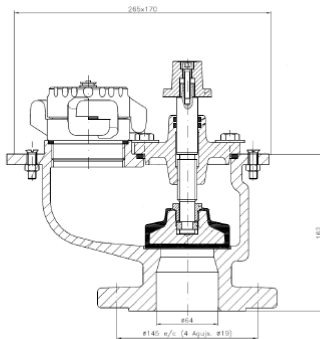
Dimensiones boca de incendios con 1 salida
