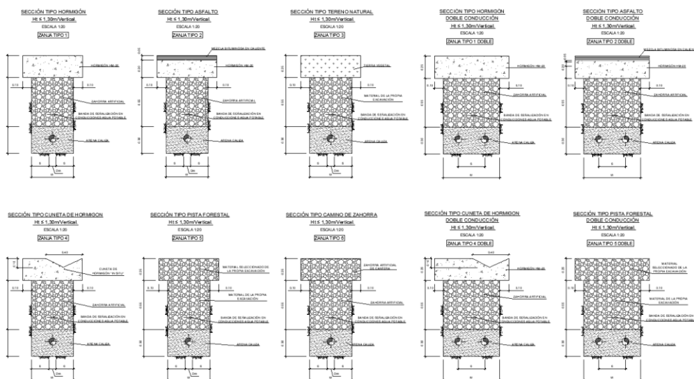
Zanjas Tipo
