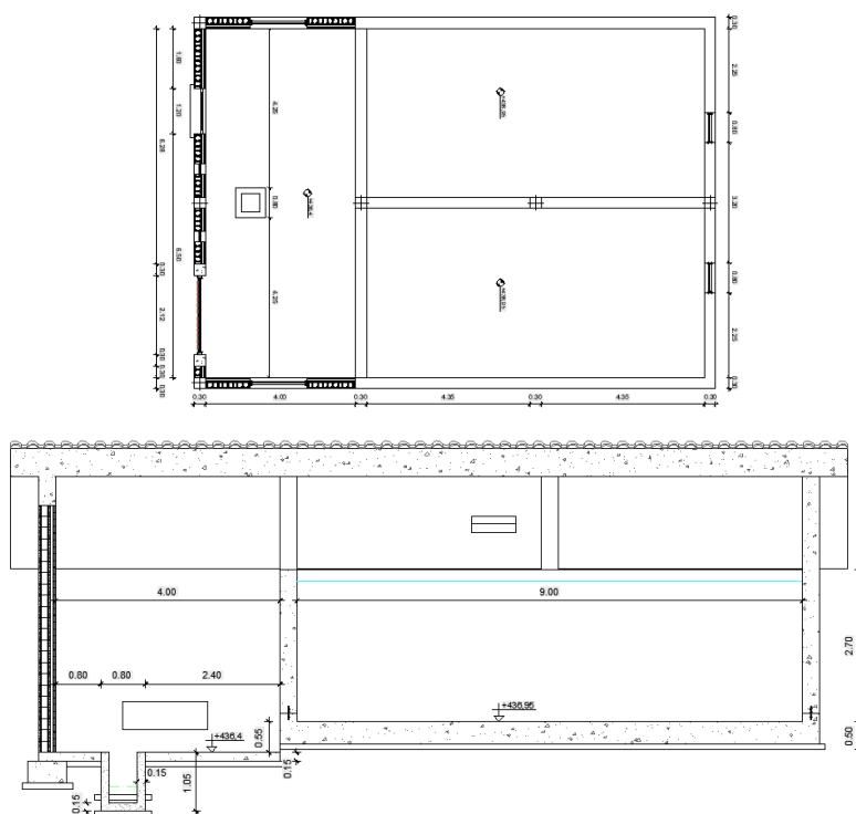
Depósito de Iturreta, implantación y geometría
