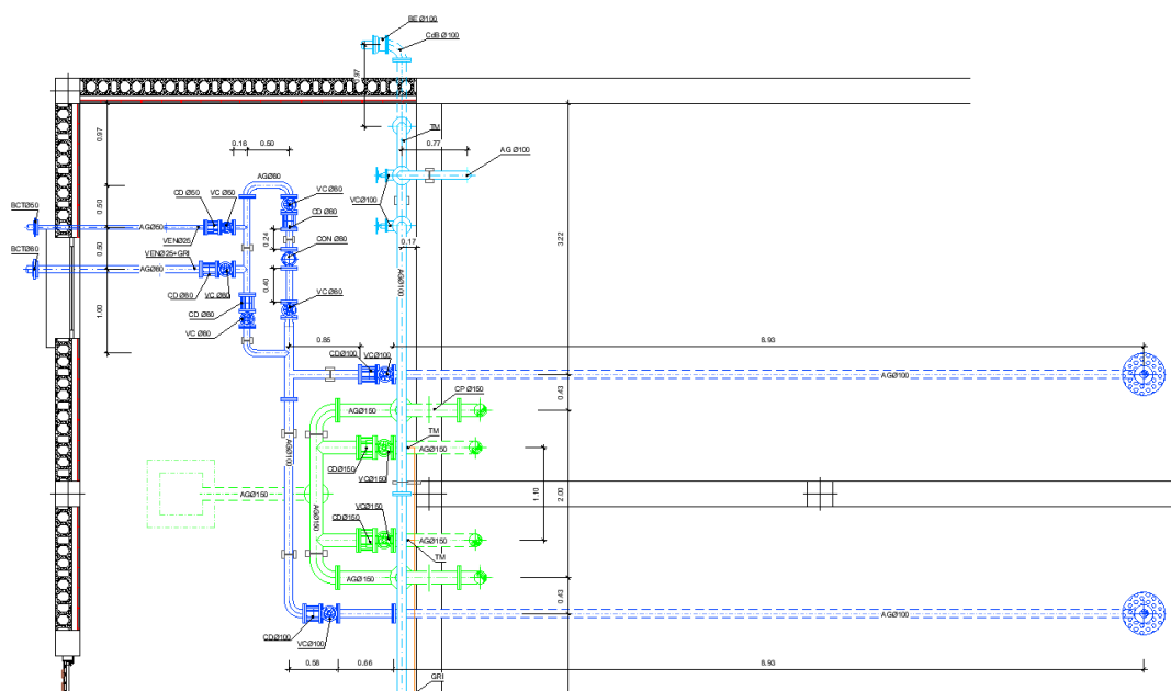
Planta de mecanismos, depósito Iturreta
