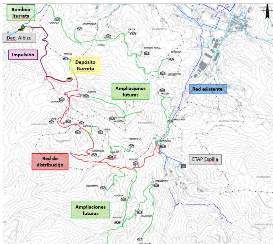
Sistema de abastecimiento de Barinaga
