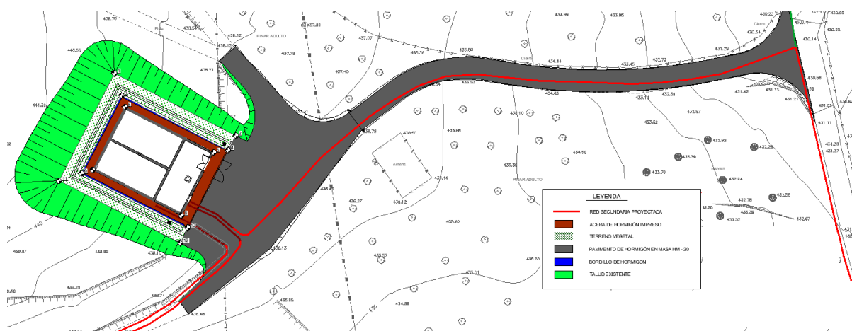
Urbanización exterior y acceso depósito de Iturreta.
