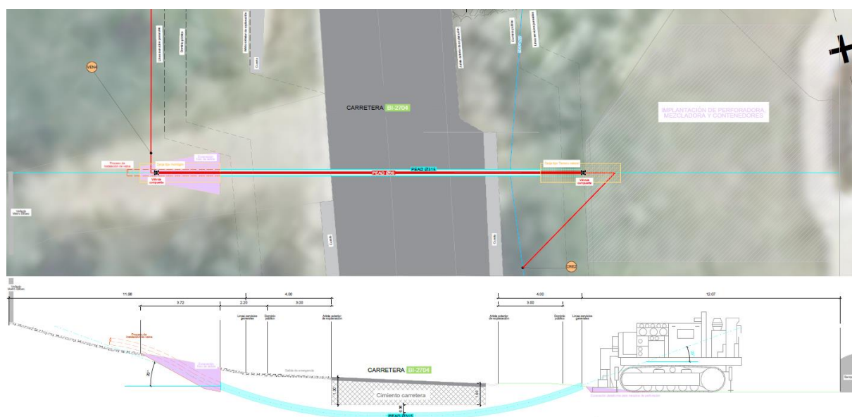
Planta y sección de la hinca horizontal dirigida
