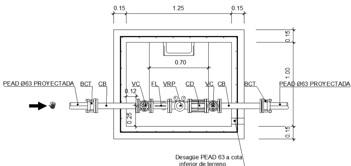
Planta de la arqueta VRP proyectada
