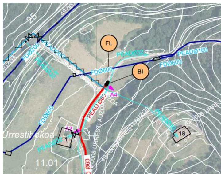
Acometida (A4), boca de incendio (BI) y final de línea (FL)
