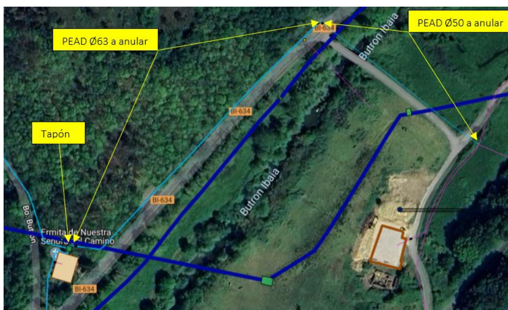
Tramos de PEAD a anular
