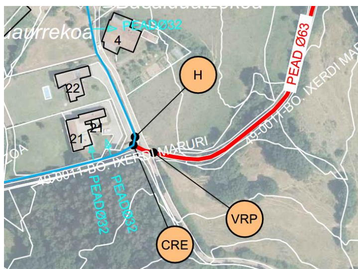
Punto de conexión a red existente (CRE) y ubicación de hidrante (H)
