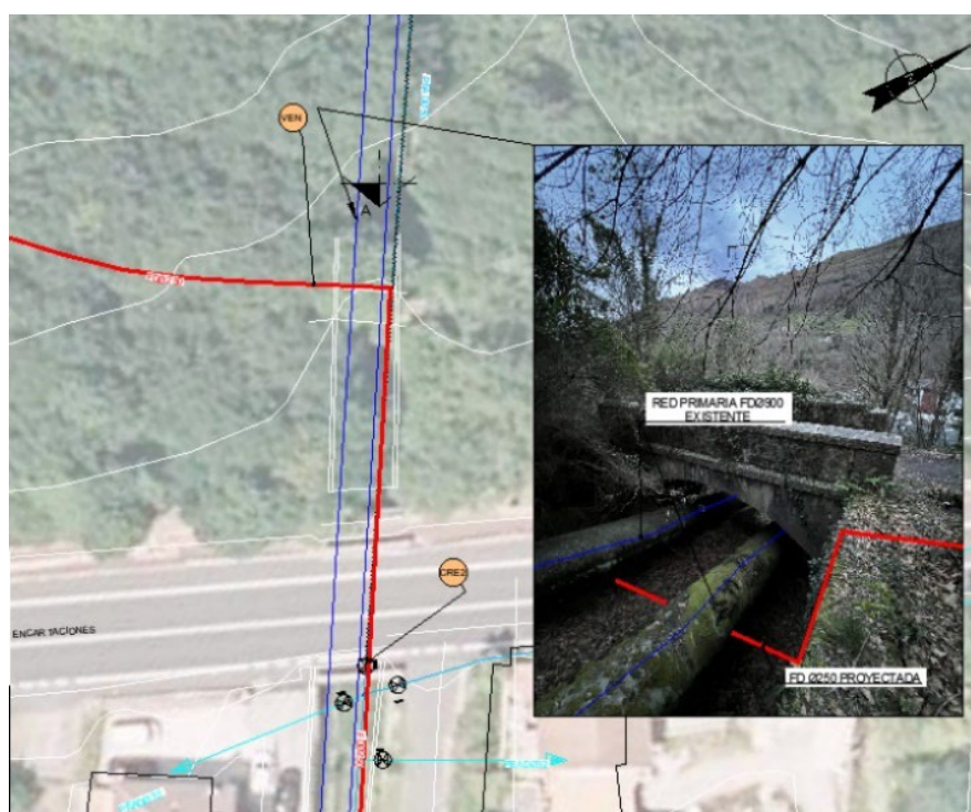
Cruce de la BI-636 por la solera del canal de Ordunte
