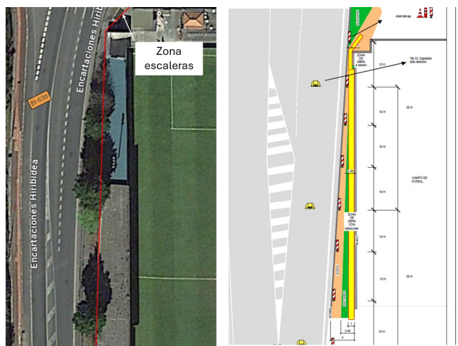
Detalle localización tubería de FD250 por el parterre del campo de fútbol de la Beluga
