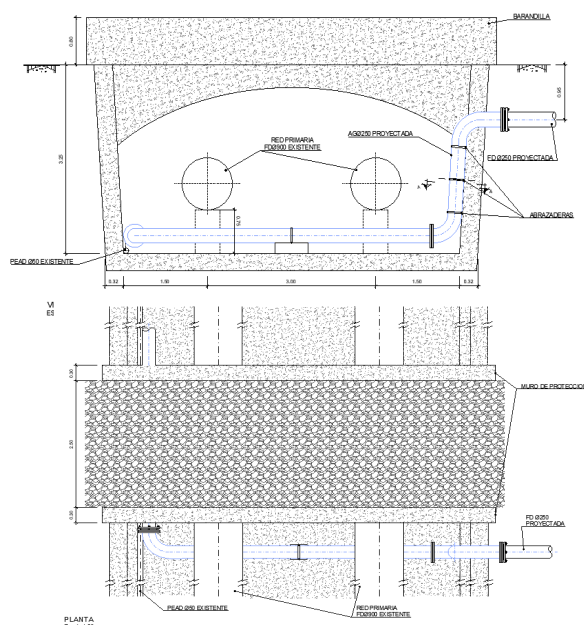
Detalle instalación de conducción en el canal de Ordunte
