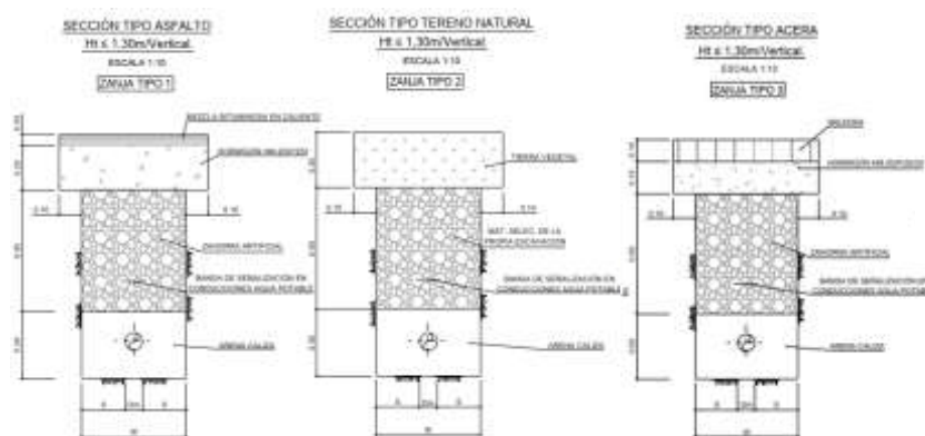
Zanjas tipo
