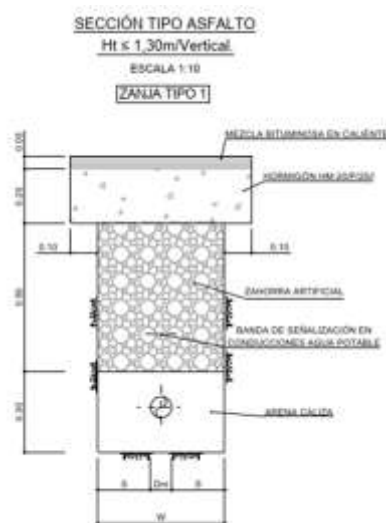
Zanjas tipo
