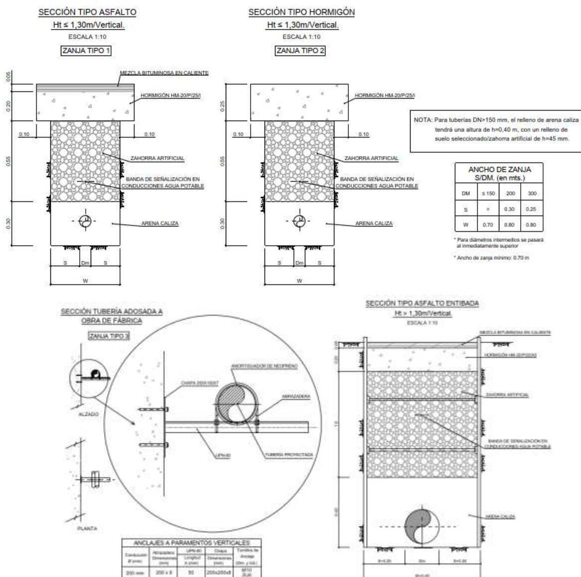
Zanjas tipo
