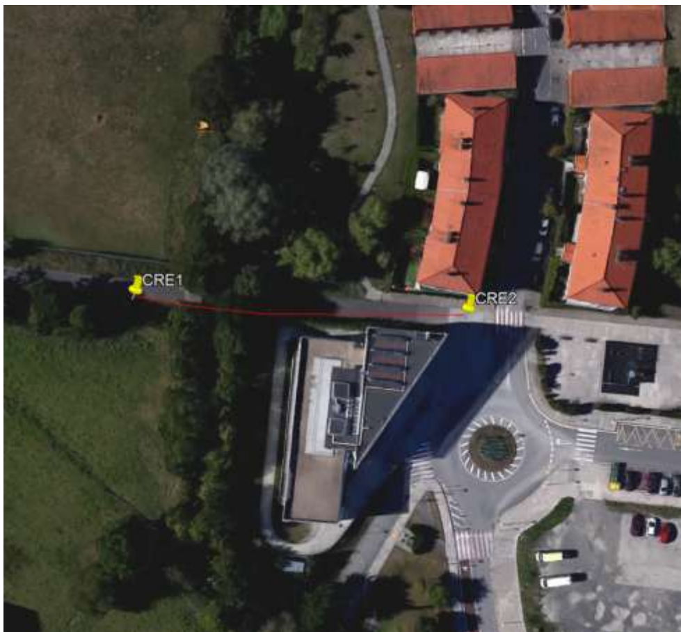
Emplazamiento de la red a ampliar en el camino San Martín de Mungia
